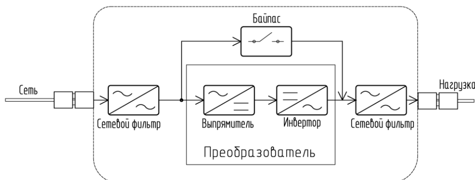
Рисунок 3 – Структурная схема принципа работы стабилизатора
