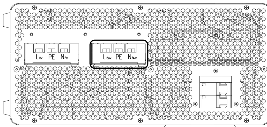
Рисунок 12в – Стабилизатор Штиль ИнСтаб IS12000. Выводы «Выход L-PE-N»
