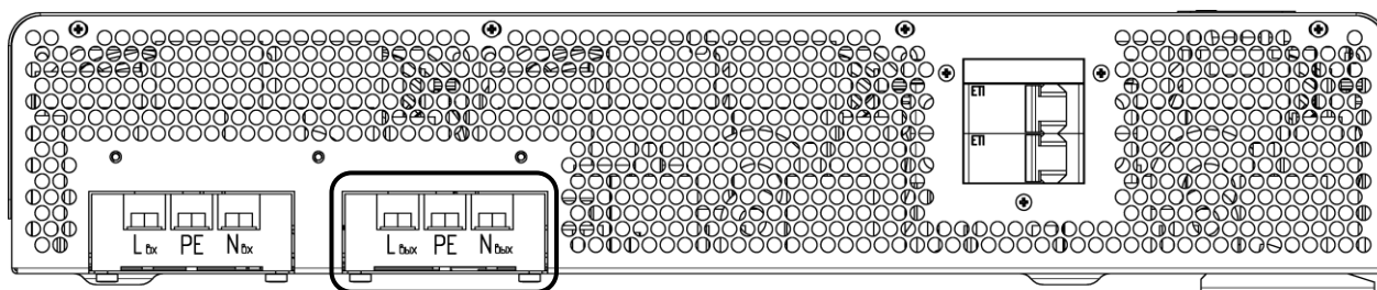
Рисунок 12б – Стабилизатор Штиль ИнСтаб IS10000. Выводы «Выход L-PE-N»
