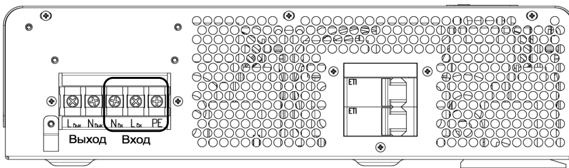
Рисунок 11а – Стабилизаторы Штиль ИнСтаб IS5000 и IS7000. Выводы «Вход N-L-PE»
