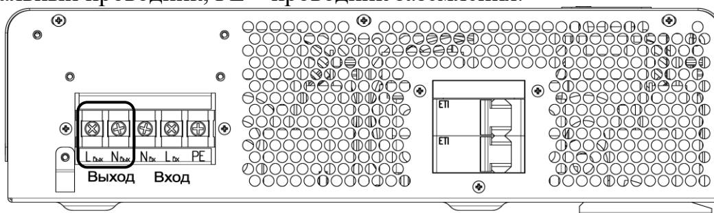
Рисунок 12а – Стабилизаторы Штиль ИнСтаб IS5000 и IS7000. Выводы «Выход L-N»
