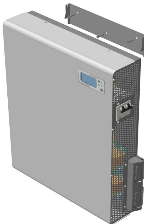
Рисунок 9б – Крепление стабилизатора Штиль ИнСтаб IS10000 на ровной вертикальной поверхности
